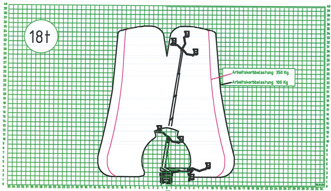
Kennfeld TKA 35,5 schmale Abstützung
