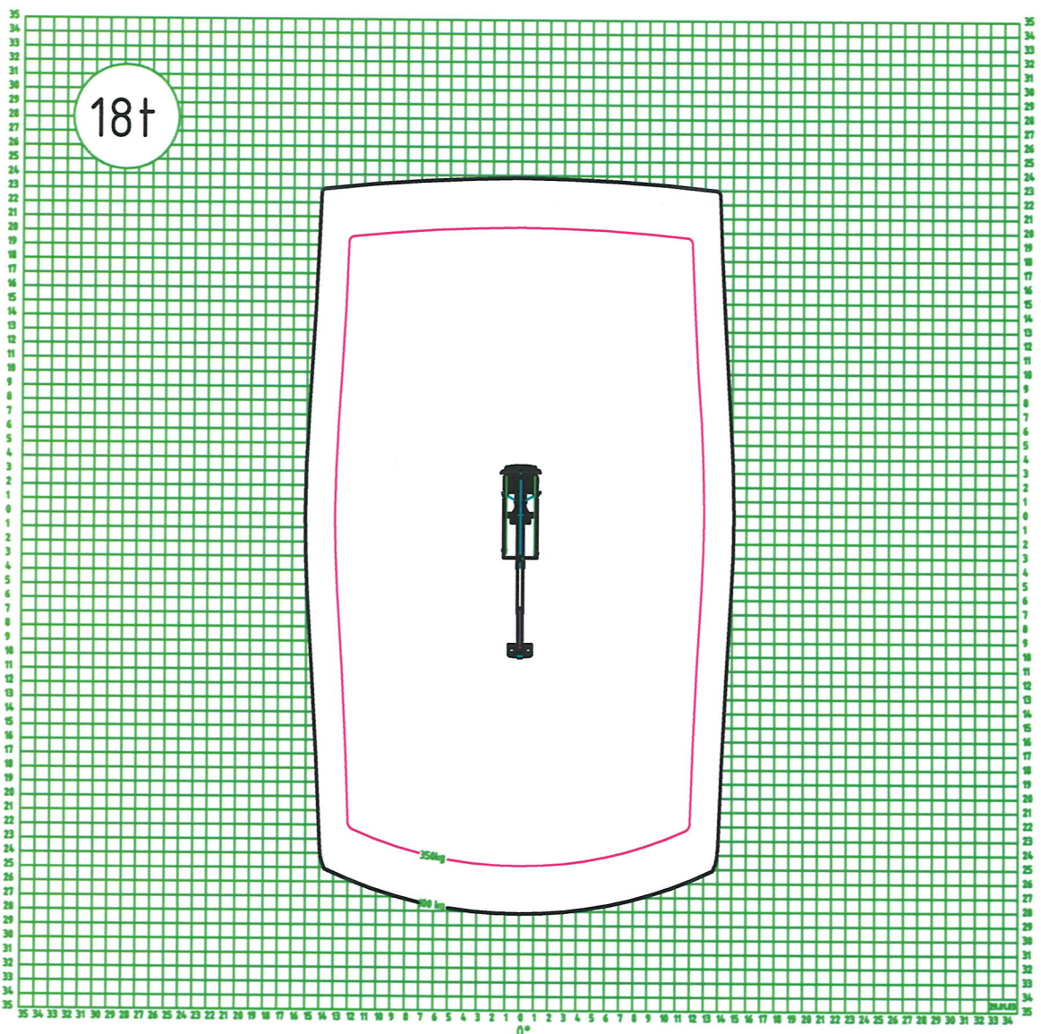
Kennfeld TKA 35,5 schmale Abstützung
