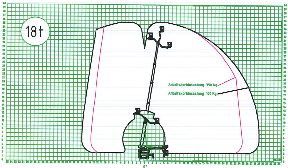
Kennfeld TKA 35,5 einseitige Abstützung
