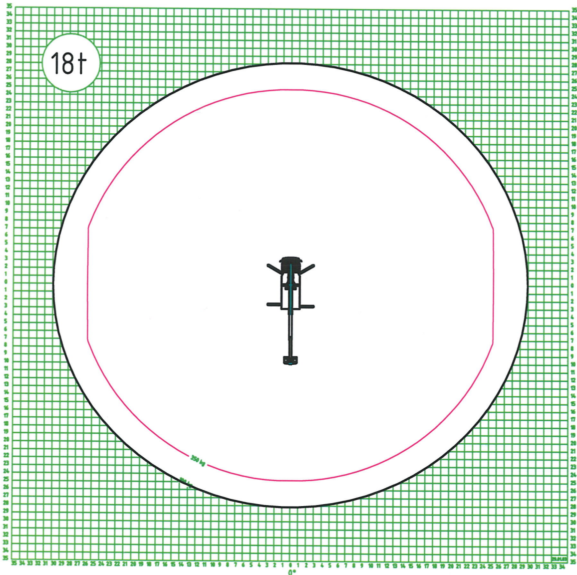
Kennfeld TKA 35,5 breite Abstützung
