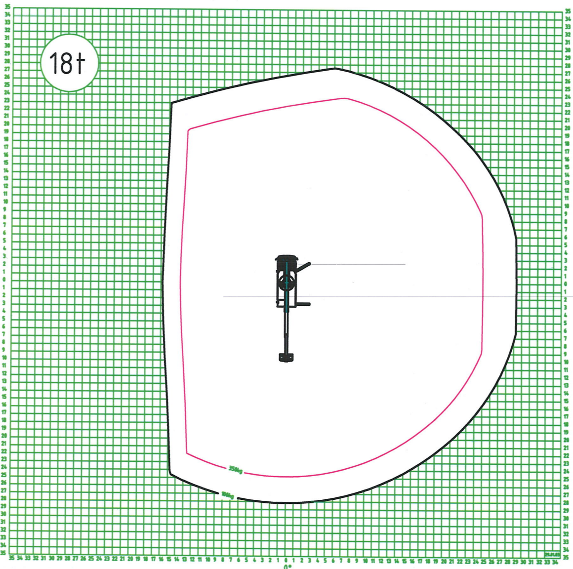
Kennfeld TKA 35,5 einseitige Abstützung
