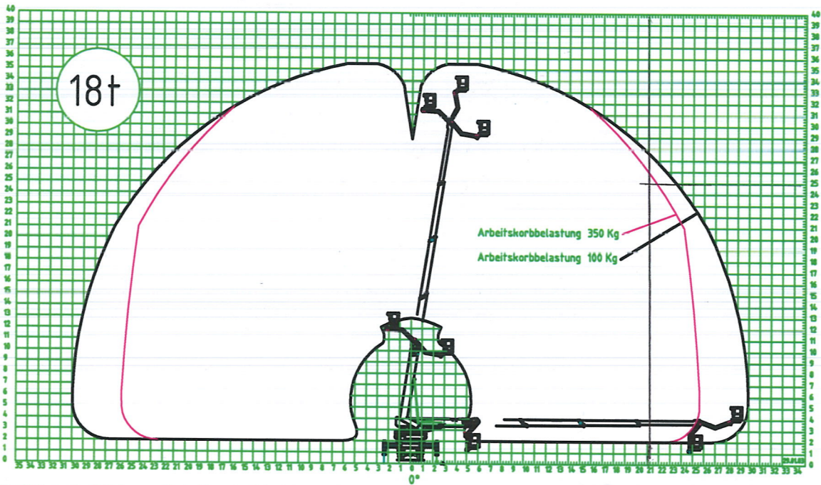
Kennfeld TKA 35,5 breite Abstützung
