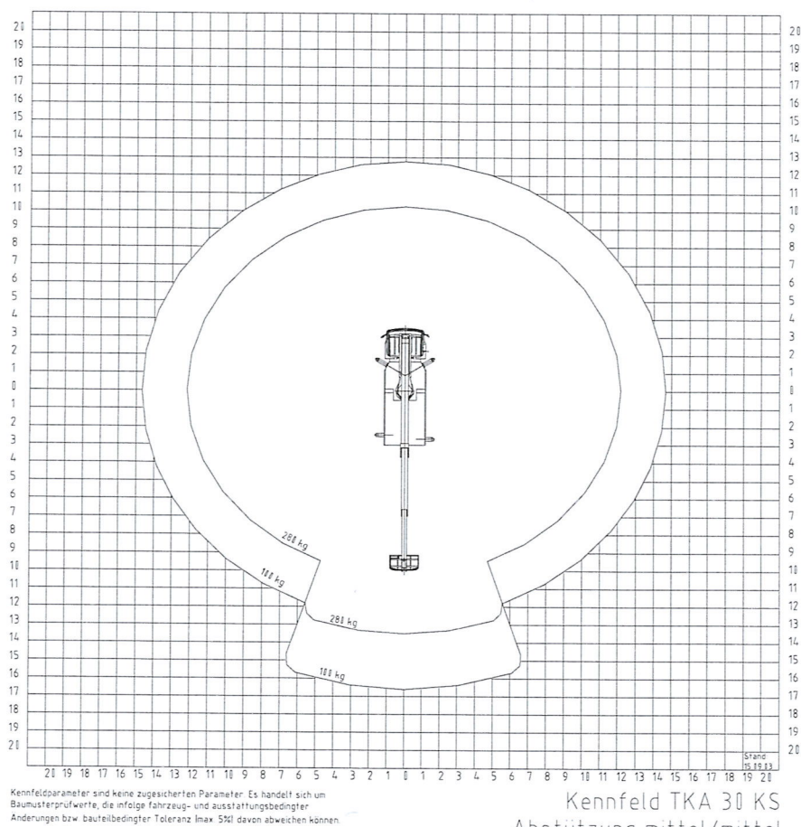
Kennfeld TKA 30 KS Abstützung mittel/mittel
